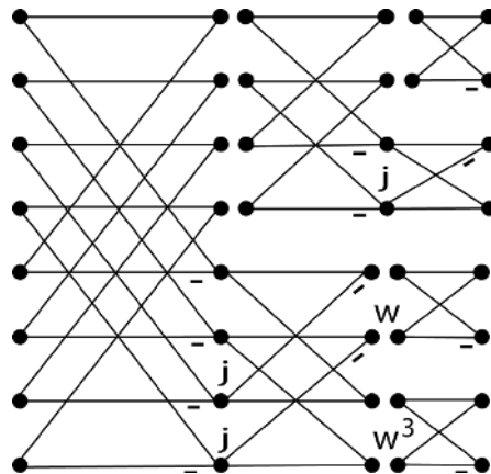
Fig. 8.4.2 Length-8 SRFFT
