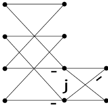
Fig. 8.4.1 SRFFT Butterfly
