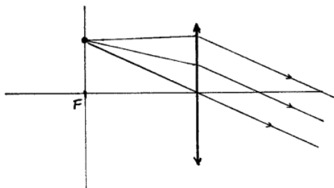
Figura 6.2.5.1: Creación de una oap (haz de rayos paralelos) mediante una lente delgada infinita y una fuente puntual monocromática. El camino óptico es reversible (reparametrización).
